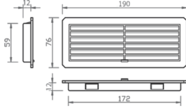
PANO KESİM ÖLÇÜSÜ 61 x 175 mm
