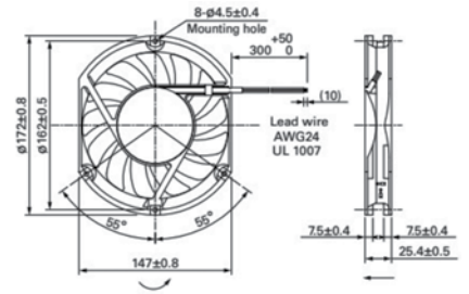
UF-DA1725B24H Ölçü : 172 x 147 x 25mm
